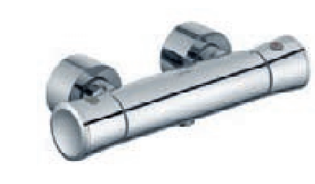
54026 Termostatická baterie pro sprchu pro nástěnnou montáž, úchyt s 50% omezením průtočného množství, bezpečnostní záračka na 38 °C, zajištěno proti zpětnému toku napojení hadice DN 15, rozteč 150 +/- 14 mm šířka: 300 mm vyložení: 110 mm
