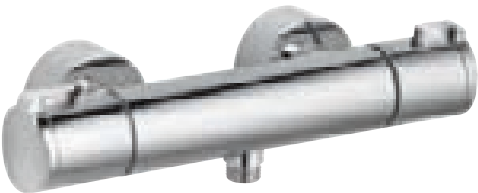
51626 Termostatická baterie pro sprchu pro nástěnnou montáž, úchyt s 50% omezením průtočného množství, bezpečnostní zarážka na 38 °C zabezpečeno proti zpětnému toku napojení hadice DN 15, rozteč 150 +/- 14 mm šířka: 307 mm vyložení: 107 mm
