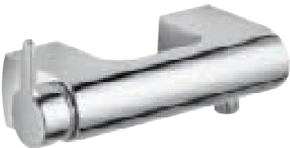
51624 Páková sprchová směšovací armatura pro montáž na zeď, směšovací kartuše s keramickými těsnicími kroužky, napojení hadice DN 15, rozteč 150 +/- 14 mm šířka: 245 mm vyložení: 97 mm
