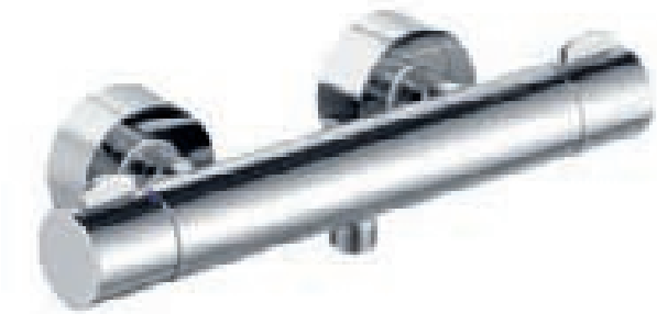
53924 Sprchová směšovací armatura DN 15 pro nástěnnou montáž keramický uzavírací ventil, směšovací ventil s keramickými těsnicími kroužky, napojení hadice DN 15, průtokové množství omezeno na 12 l/min, rozteč 150 +/- 14 mm šířka: 311 mm vyložení: 104 mm
