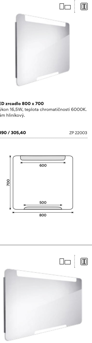
LED zrcadlo 1200 x 700 Výkon 28,5W, teplota chromatičnosti 6000K. Rám hliníkový.
