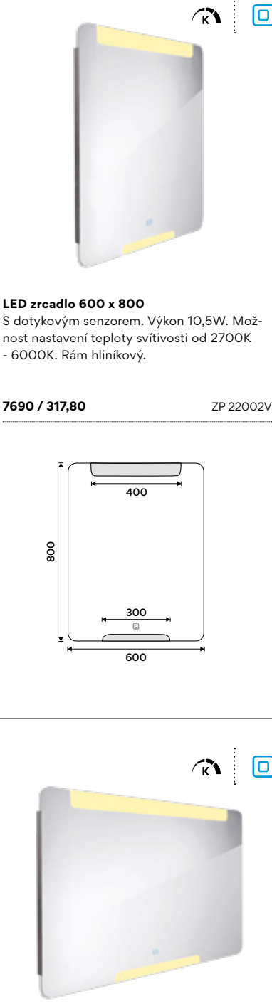
LED zrcadlo 1000 x 700 S dotykovým senzorem. Výkon 22,5W. Mož- nost nastavení teploty svítivosti od 2700K - 6000K. Rám hliníkový.
