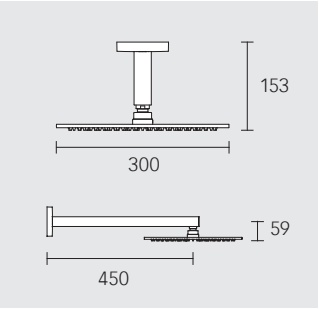
Hlavová sprcha
