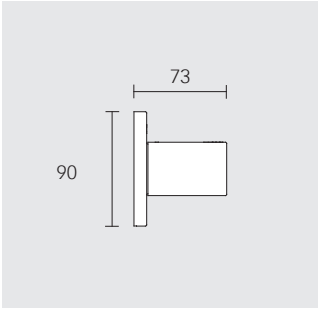
3cestný podomítkový přepínací ventil DN 15
