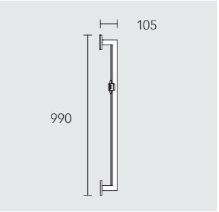
Sprchová tyč
