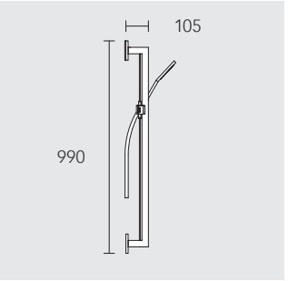
Sprchová sada
