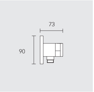
Napojení hadice s držákem sprchy DN 15
