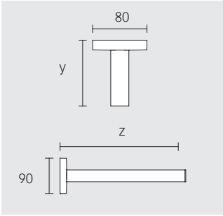
Rameno sprchy DN 15
