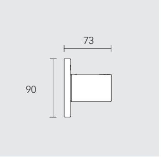
2cestný uzavírací a přepínací ventil Instalace pod omítku DN 15
