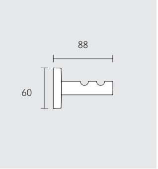
Háček na ručník dvojitý
